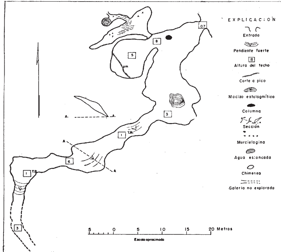
CUEVA DEL AIRE, HUICHIHUAYAN, S. L. P. Plano esquemático
