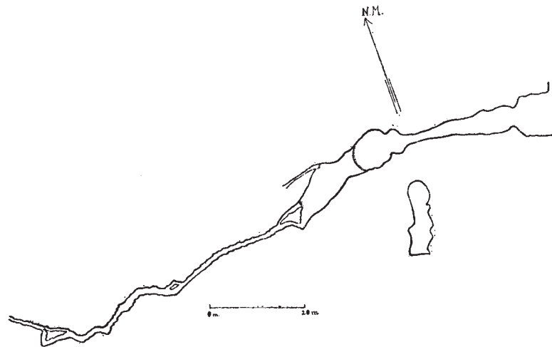
Fig. 8.—Plano esquemático de la Cueva de Taninul n. 1. Desarrollo a lo largo de una diaclasa. Etapa de madurez.
