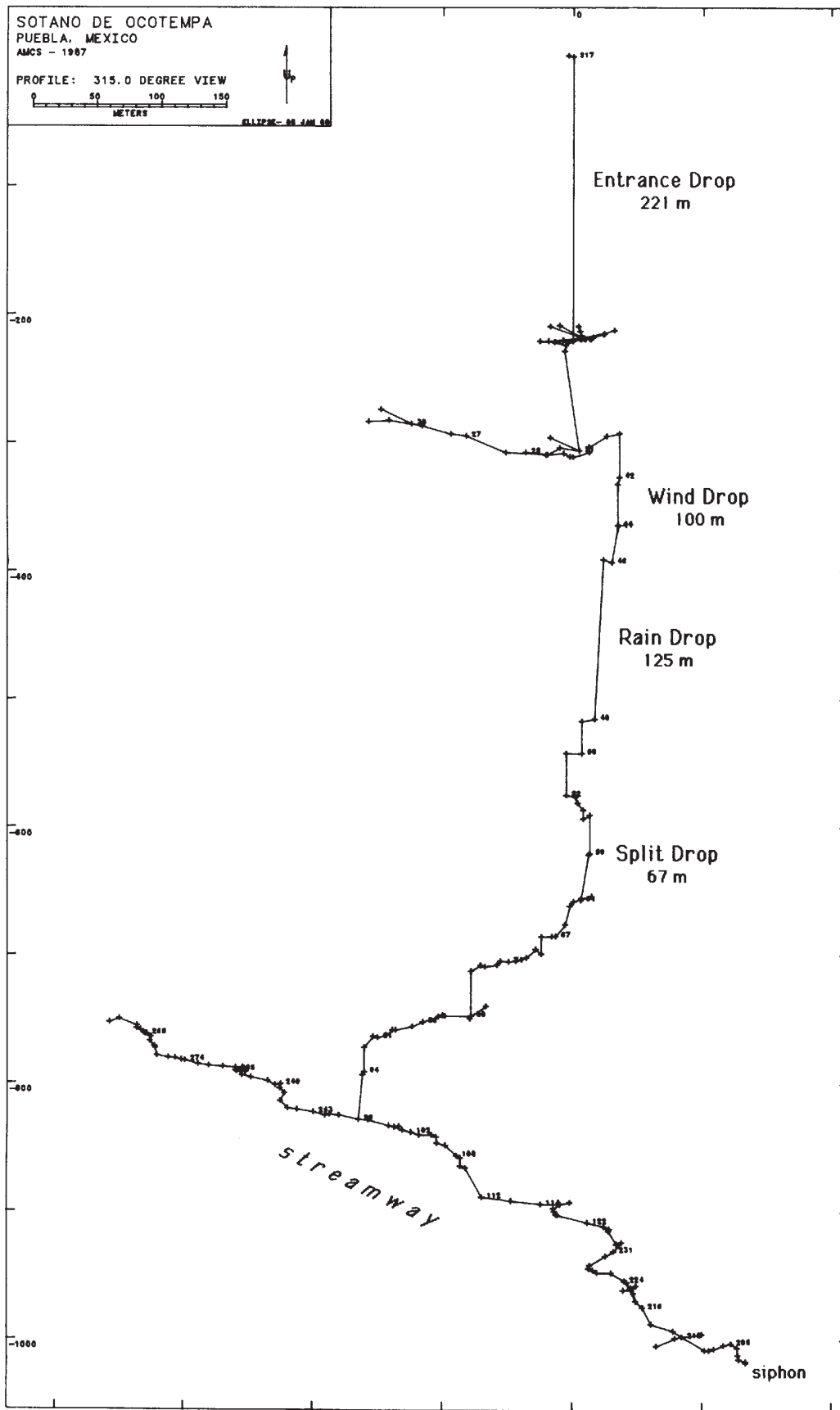
Sótano de Ocotempa Ocotempa, Mpo. Ajalpan Puebla Texas Caver, v. 32, no. 6, p. 149, 1987
