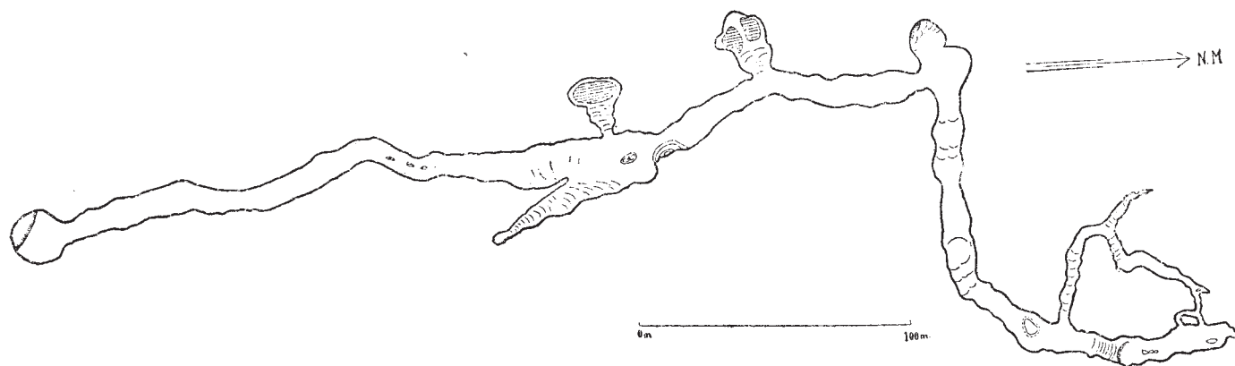
Fig. 1.—Plano esquemático de la Cueva de Quintero. Obsérvense las direcciones N-S y E-W predominantes en la galería principal según las diaclasas; los dos divertículos con lagunas permanentes están a más bajo nivel que la galería; en la cámara del centro hay grandes estalagmitas. Etapa de madurez.
