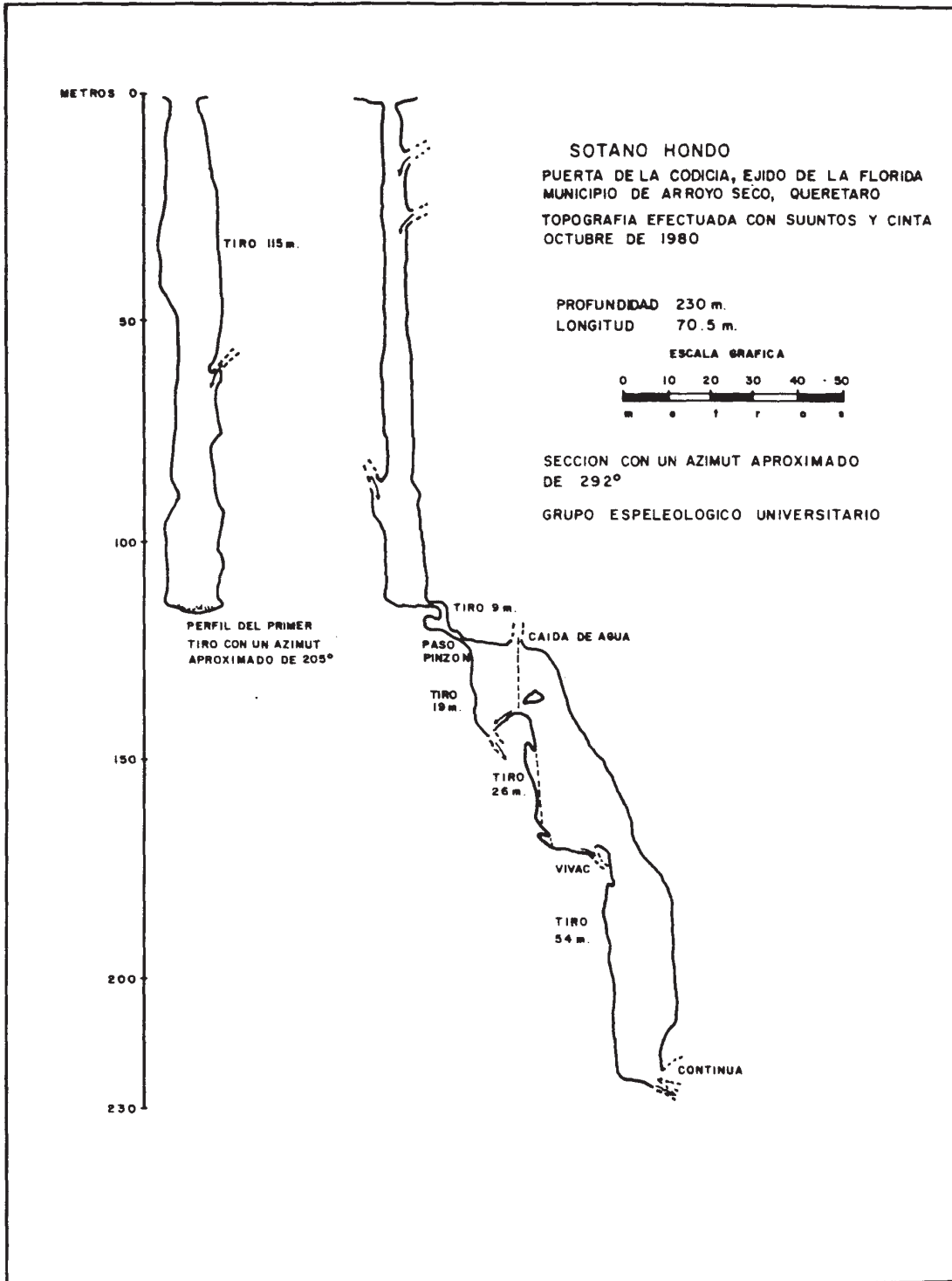
Sótano Hondo La Florida, Mpo. Arroyo Seco Querétaro Las Cavernas de la Sierra Gorda, v. 1, p. 127, 1986
