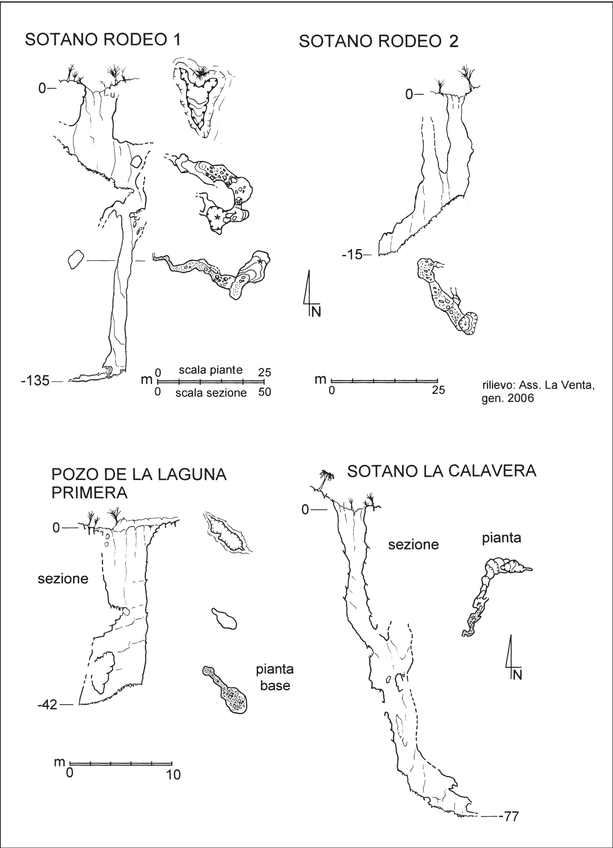
Sótano Rodeo 1, Sótano Rodeo 2, Pozo de Laguna Primera, Sótano la Calavera Mpo. Santa María Ixcatlán Oaxaca
