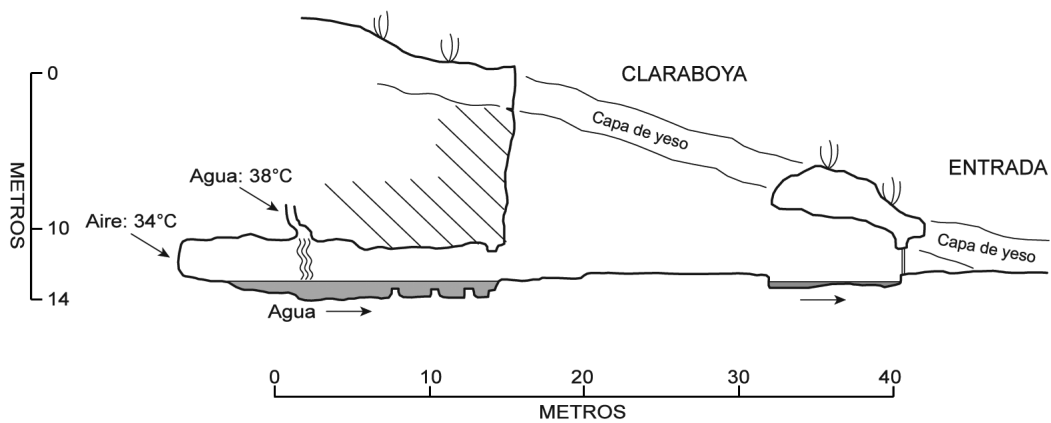
VISTA PERFIL: 130°
