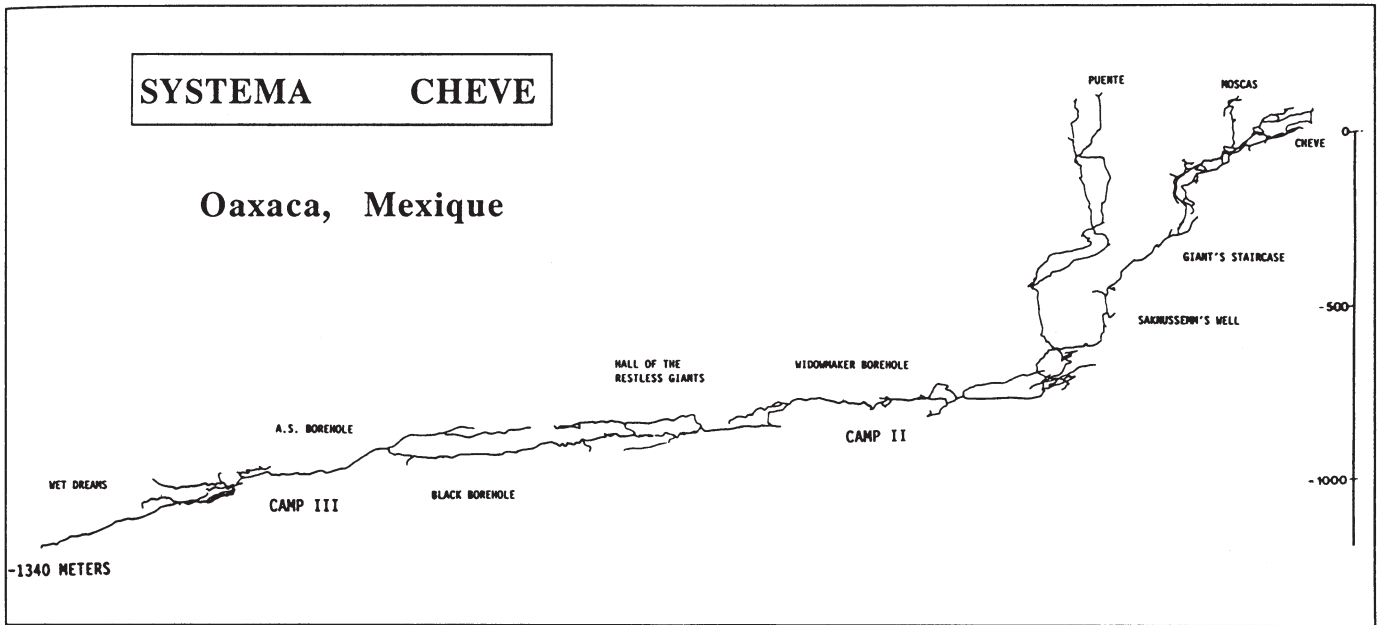
Coupe projetée du Sistema Cheve tel qu'il se présentait fin 1990. (d'après COONS & KAMBESIS, 1991)
