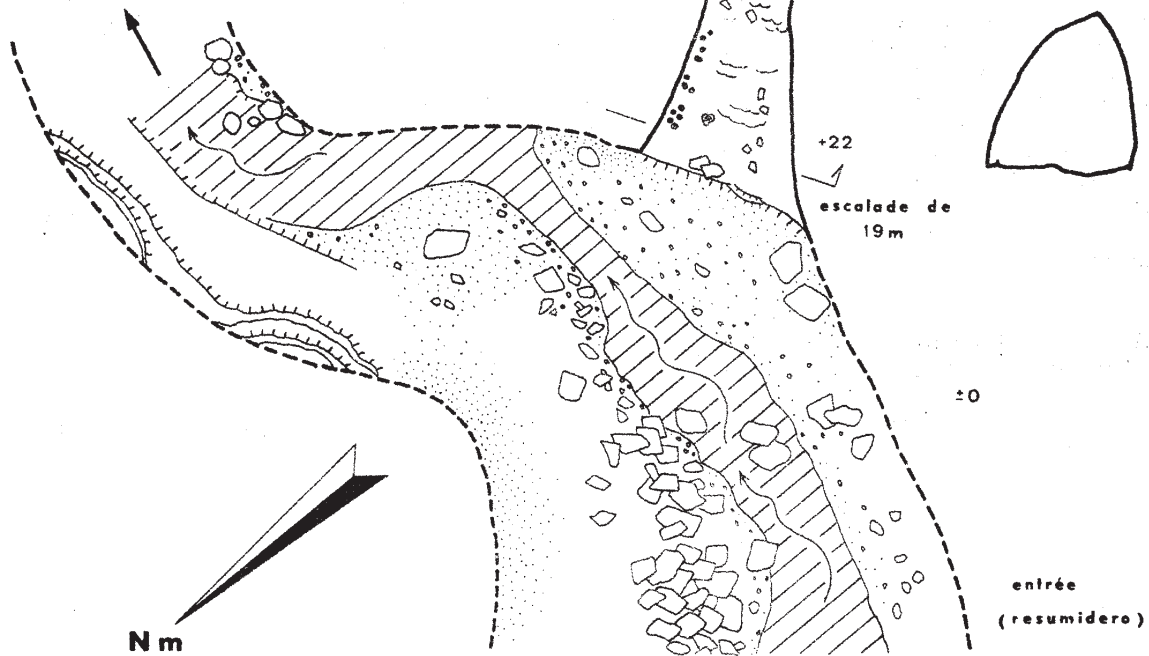
Río Subterráneo de Chontalcoatlán Cacahuamilpa, Mpo. Picaya Guerrero Grottes et Gouffres no. 76, p. 8, 1980
